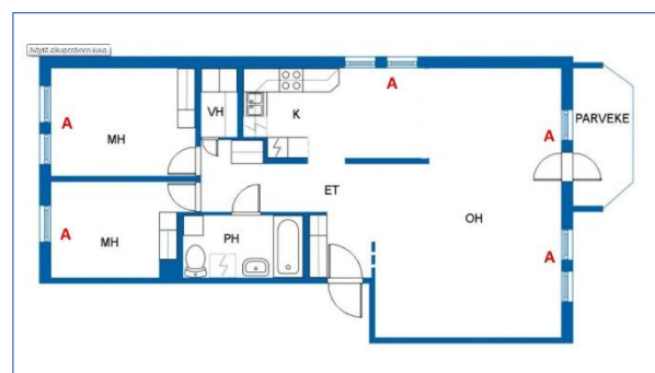
Kuva 3 Kuvassa esimerkki ikkunaan integroitujen antennien sijainnista kerrostalokolmiossa (A = antenni ikkunassa). Kuvassa minimimäärä antennia per huoneisto. Piirustuksiin yksilöidään esim. F1/ANT. Antenni sijaitsee ikkunayksikössä pystysivulla vasemmassa reunassa.
