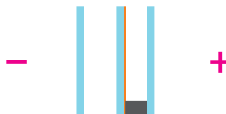
Ikkunan ulkopuitteessa tasolasi, sisäpuitteessa kaksinkertainen eristyslasi.
